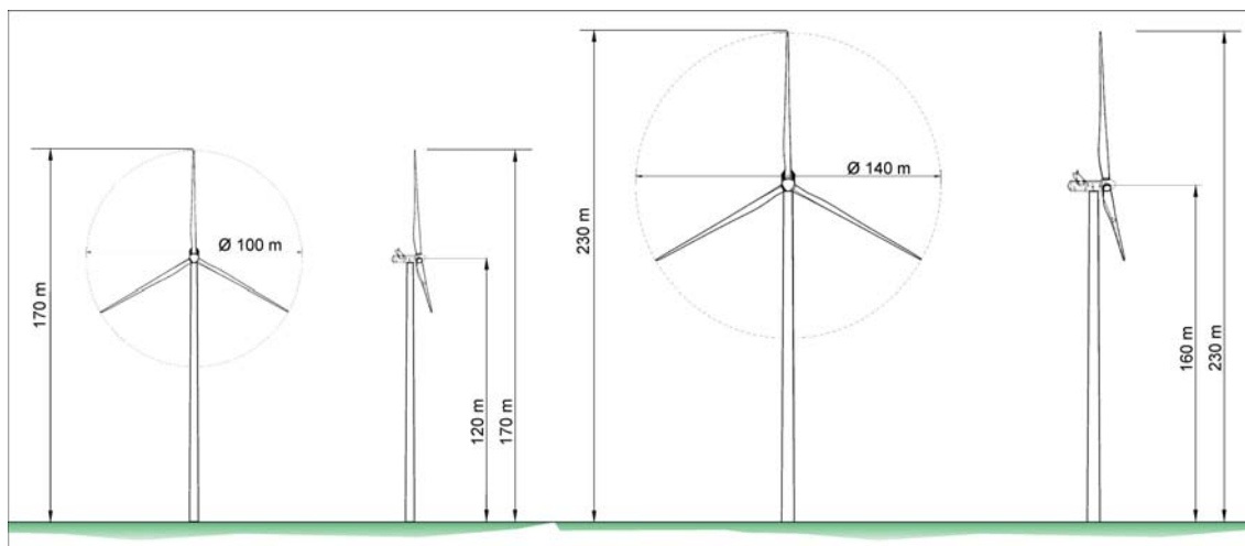
Kuva 31. Mallikuvat voimalakorkeuksista.
