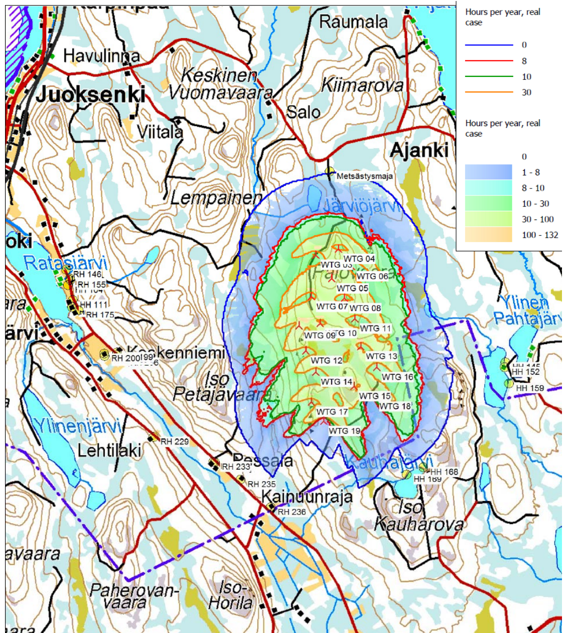
Kuva 50. Varjostusmallinnuksen tulokset (real case).
