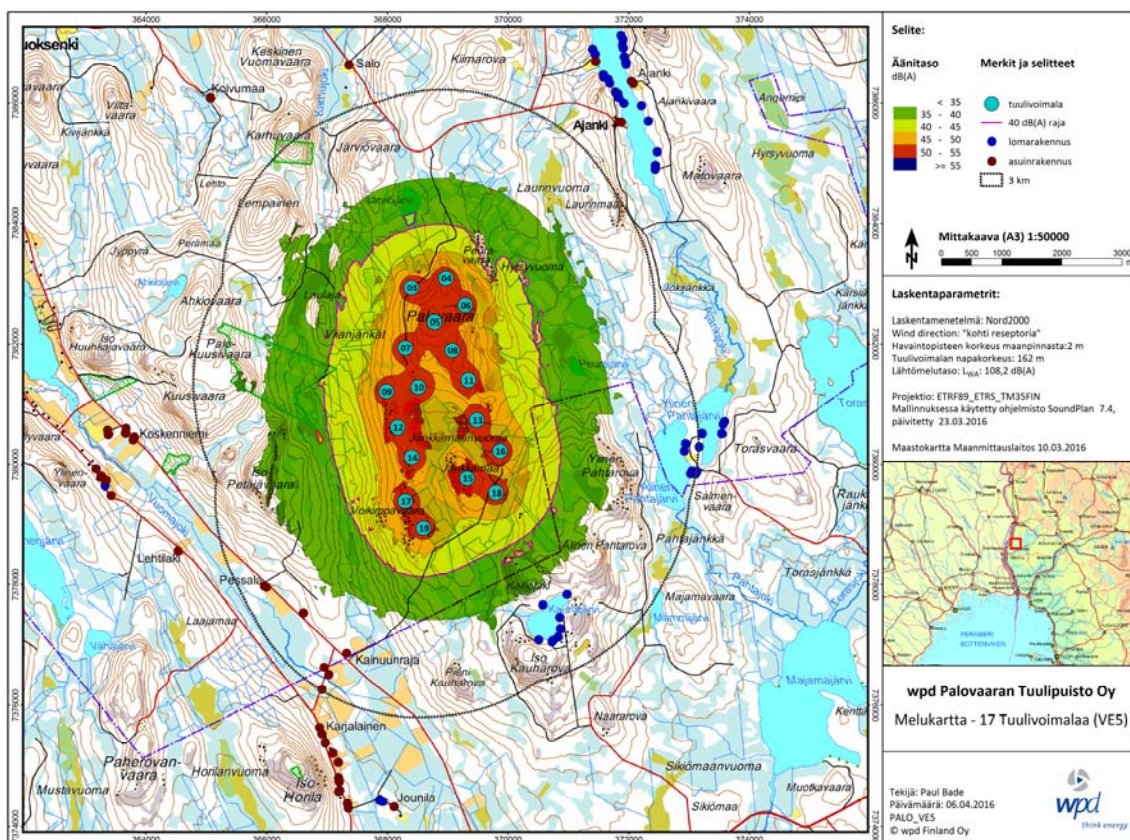
Kuva 48. Melumallinnuksen tulokset (Nord 2000).
