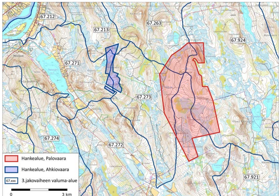
Kuva 16. Tuulivoimapuistoalueiden sijoittuminen 3. jakovaiheen valuma-alueille (Oiva 2014). Palovaaran alue on punaisella värillä. Aluerajaus kuvassa on YVA-vaiheen mukainen.
