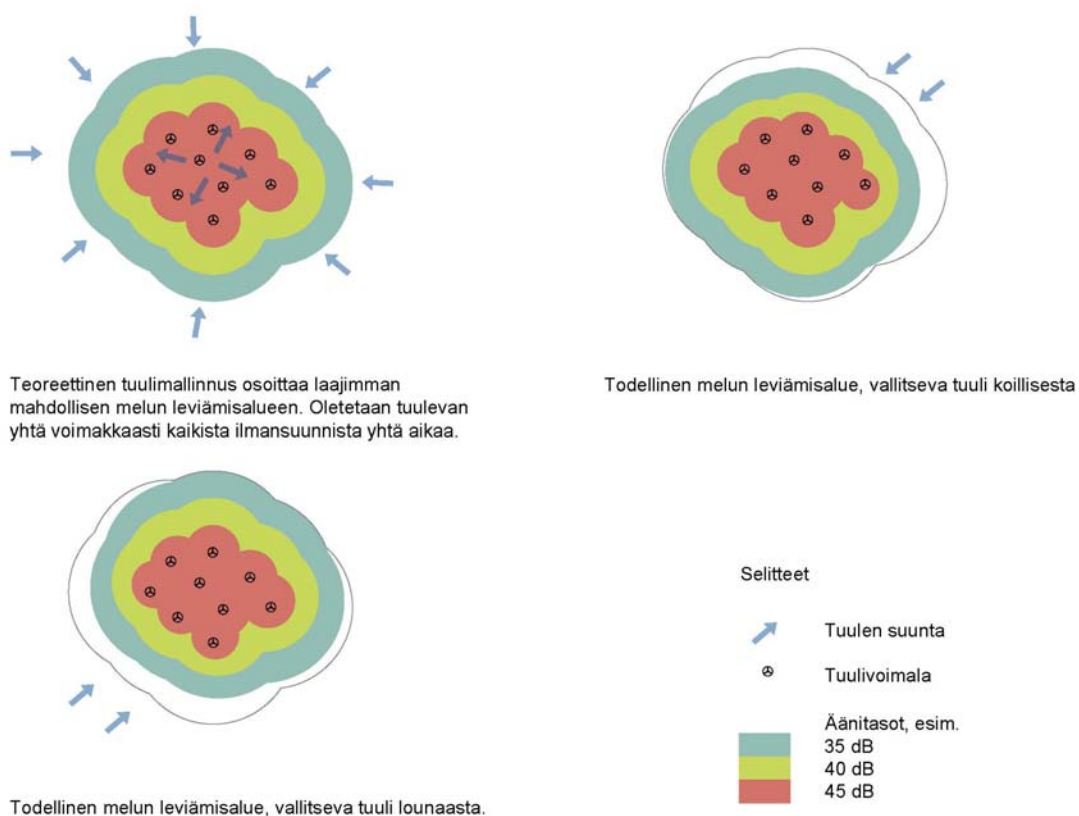
Kuva 47. Mallikuva teoreettisesta melumallinnuksesta ylhäällä ja todellisen ti-lanteen mukaisesta tuulivoima-melun leviämisestä alhaalla.
