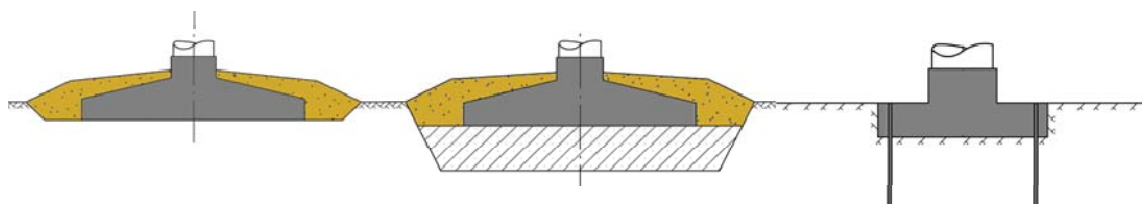
Kuva 32. Tuulivoimalat voidaan perustaa useilla eri tavoilla. Periaatekuvat maanvaraisesta teräsbetoniperustuksesta, teräsbetoniperustuksesta massanvaih-dolla sekä kallioankkuroidusta teräsbetoniperustuksesta.
