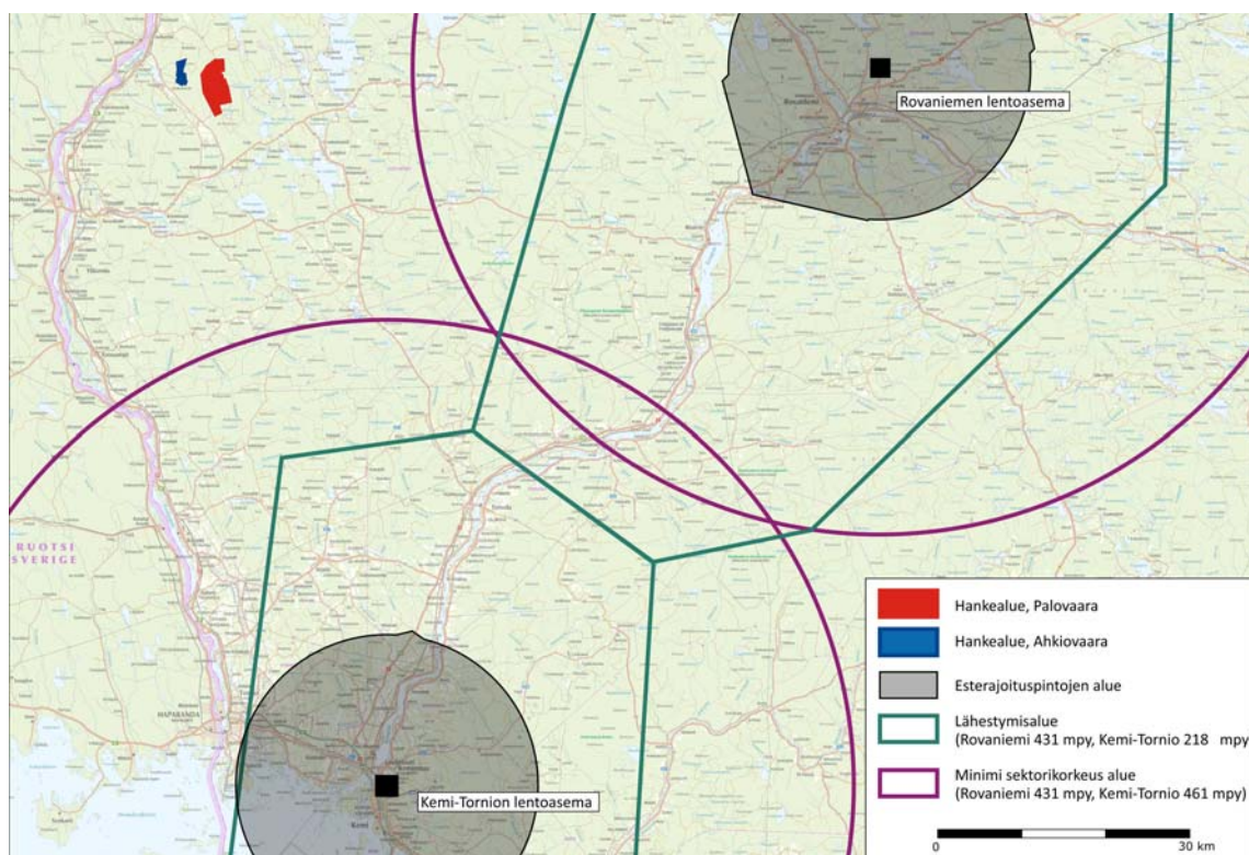
Kuva 10. Palovaaran ja Ahkiovaaran tuulivoimapuistojen sijoittuminen suhteessa Rovaniemen ja Kemi-Tornion lentoasemien korkeusrajoitusalueisiin. Palovaaran alue on punaisella värillä. Aluerajaus kuvassa on YVA-vaiheen mukainen, Ahkiovaaran alueesta on luovuttu.
