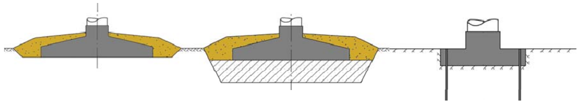
Kuva 32. Tuulivoimalat voidaan perustaa useilla eri tavoilla. Periaatekuvat maanvaraisesta teräsbetoniperustuksesta, teräsbetoniperustuksesta massanvaih-dolla sekä kallioankkuroidusta teräsbetoniperustuksesta.
