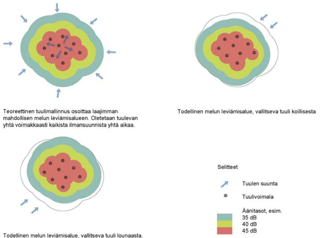
Kuva 48. Mallikuva teoreettisesta melumallinnuksesta ylhäällä ja todellisen ti-lanteen mukaisesta tuulivoima-melun leviämisestä alhaalla.
