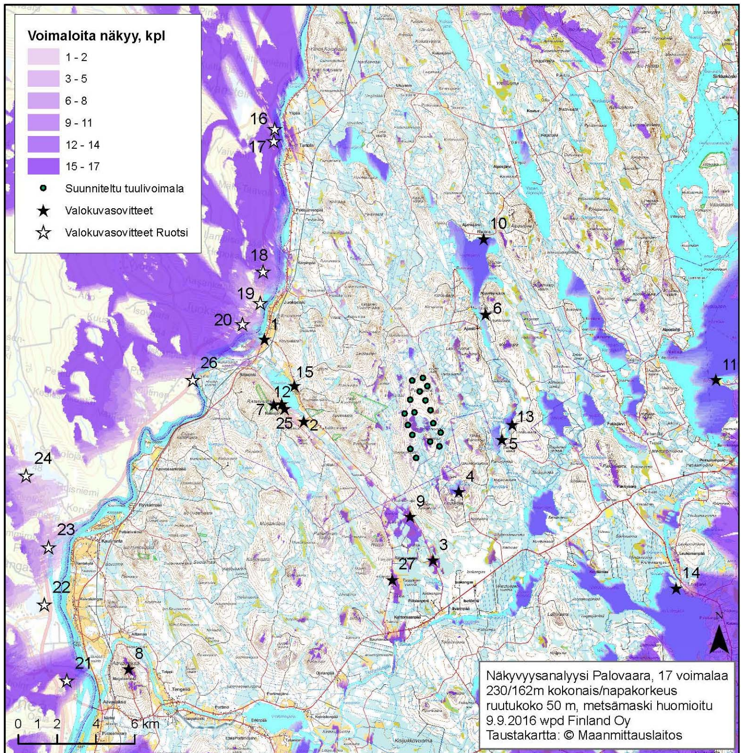
Kuva 37. Näkymäanalyysikartta. Voimaloiden napakorkeus on 162 metriä ja kokonaiskorkeus 230 metriä. Valokuvasovitteiden ottopaikat on esitetty tähdillä.
